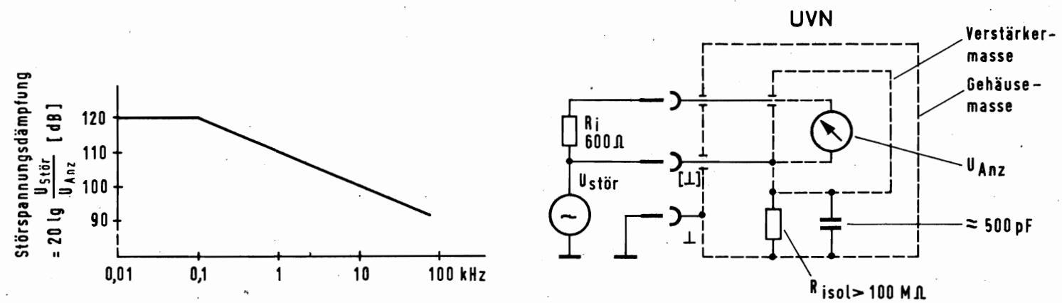
Bild 1. Frequenzabhängigkeit der Störspannungsdämpfung bei R_i = 600 \Omega
