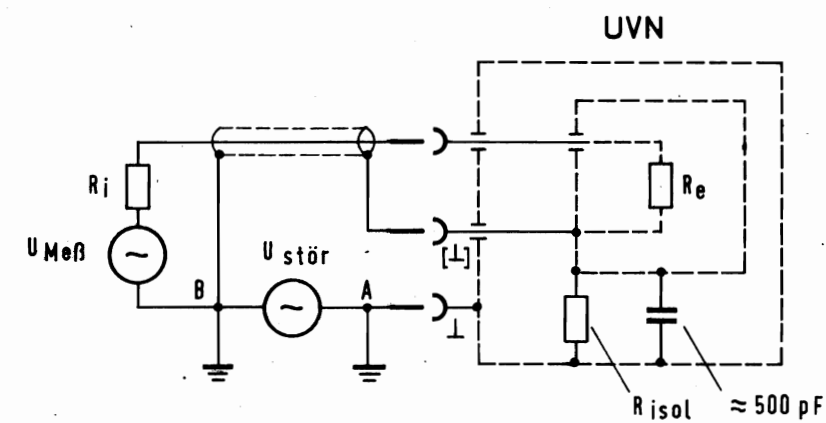
Bild 2. Unterdrückung der Störspannung U_{stör} durch den erdfreien Aufbau des Verstärker- und Anzeigeteils
